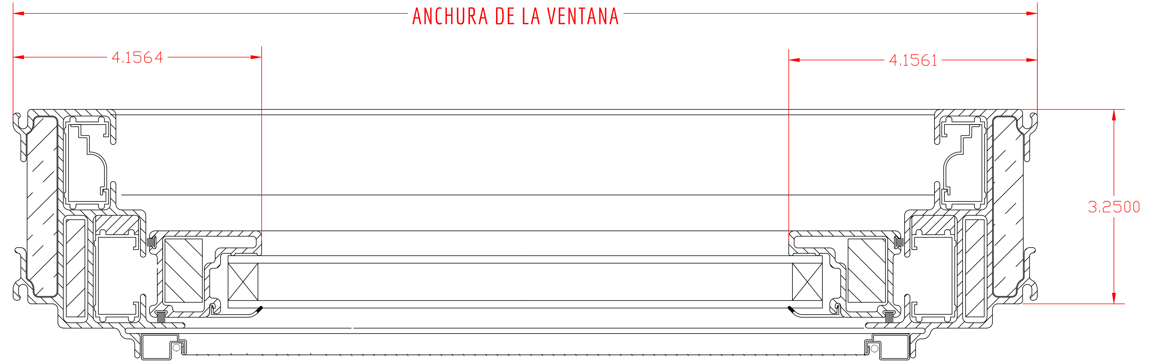
PARTE SUPERIOR DEL MARCO DE GUILLOTINA
